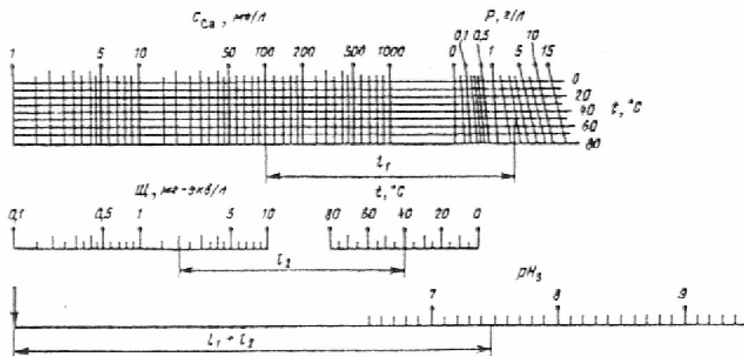
Рис. 1. Номограмма для определения рН насыщения воды карбонатом кальция (рНс)
